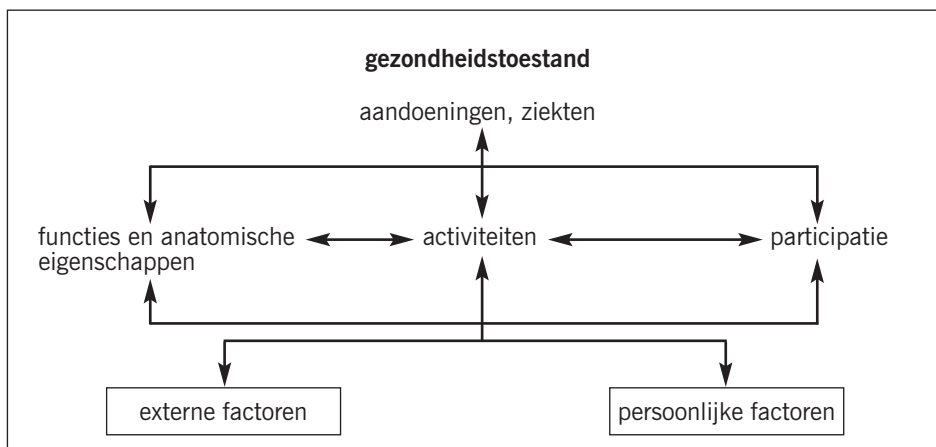
Figuur 3. ICF-model 1
